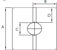
Abdeckblende 46°-55°
