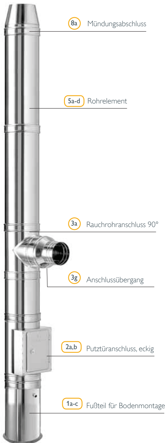
Bodenmontage
