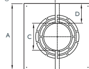
Abdeckblende 30° - 45° für Hinterlüftung
