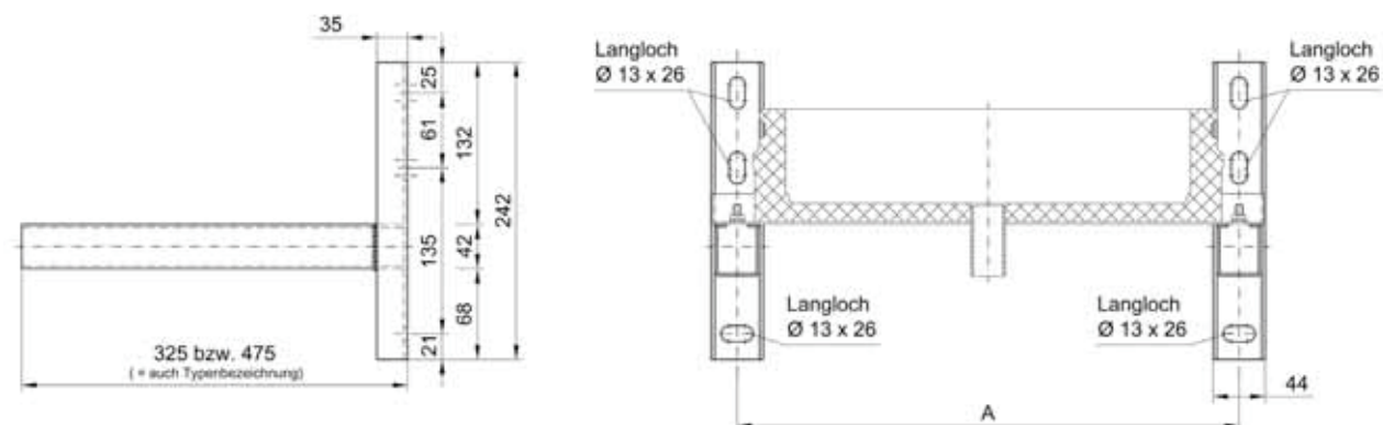
Montagemaße Wandmontage bei "Verlängerter Wandkonsole" Typ 570 bis Typ 1304
