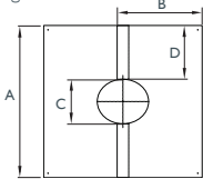
Abdeckblende 56°-60°
