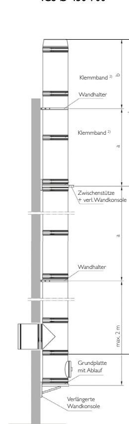
ICS Ø 450-700
