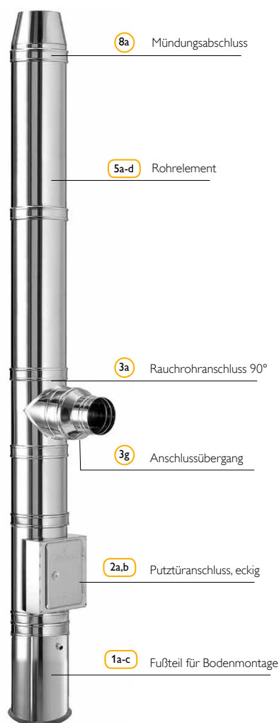
Bodenmontage
