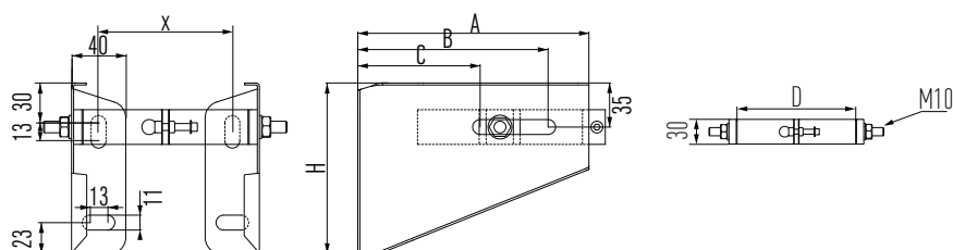
Wandstütze Paar für Wandabstand 90-200 mm inkl. USMO / Stützband
