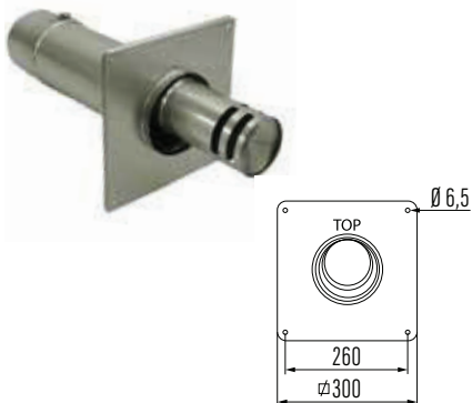
Horizontale Mündung 100 exzentrisch mit Abdeckblende eckig 300
