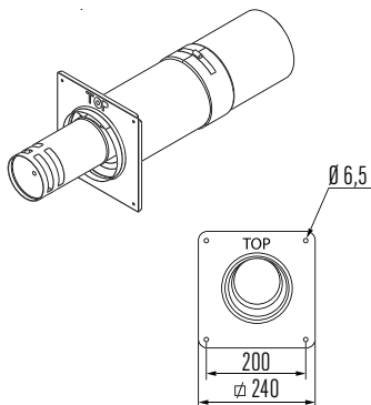
Horizontale Mündung 100 exzentrisch Typ USDHC1 mit Abdeckblende eckig 240
