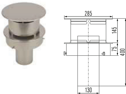
Mündungsabschluss mit Regenhaube und Windabweiser
