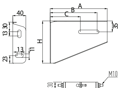
Wandstütze (Paar) für Wandabstand 90-200 mm inkl. UEMO / Stützband
