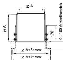
LB90 – Wandhalter
