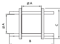
LB90 – Sparrenhalter (Einzelteile lose gepackt)
