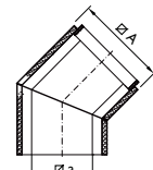
LB90 – Bogen 45°
