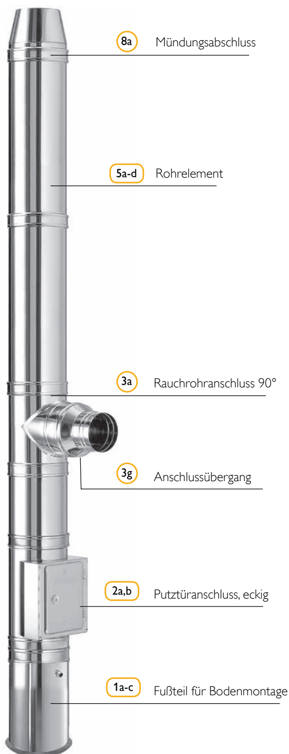
Bodenmontage
