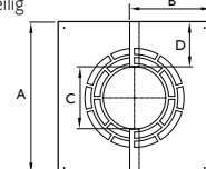
Abdeckblende 30° - 45° für Hinterlüftung *
