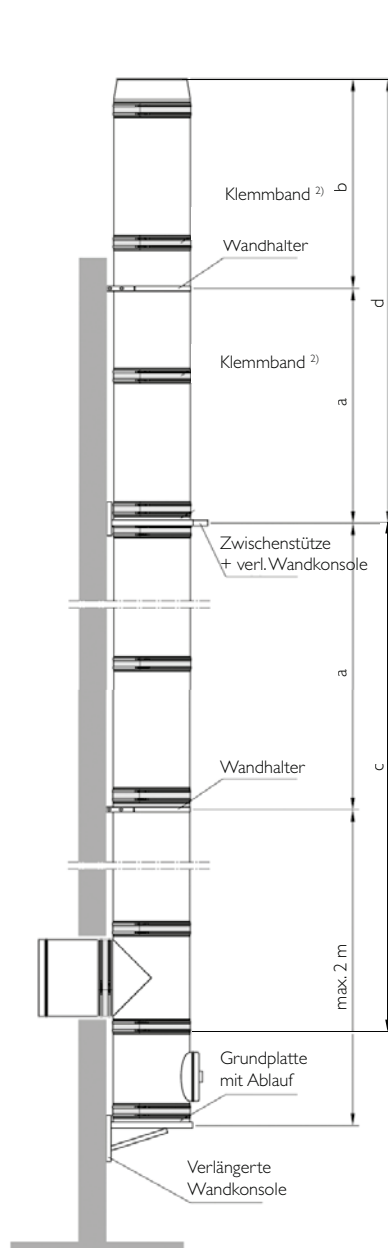
ICS Ø 450-700
