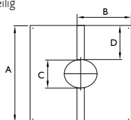
Abdeckblende 0° - 30° für Hinterlüftung
