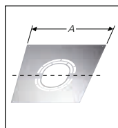
Abdeckblende 30° - 45° für Hinterlüftung *
