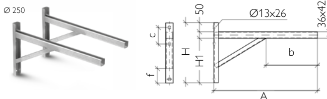
Verlängerte Wandkonsole (Paar) bis 400 mm Art.-Nr. alt UEOH4
