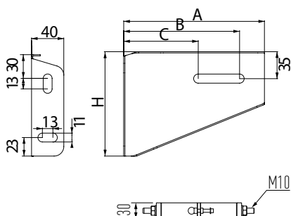
Wandstütze (Paar) für Wandabstand 90-200 mm inkl. UEMO / Stützband Art.-Nr. alt UEO 2
