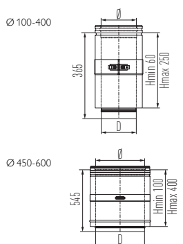
Längenausgleichselement
