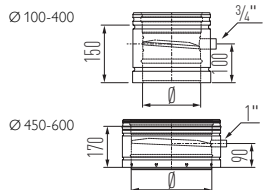
Entwässerungselement, senkrecht
