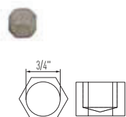
Verschlusskappe 3/4"
